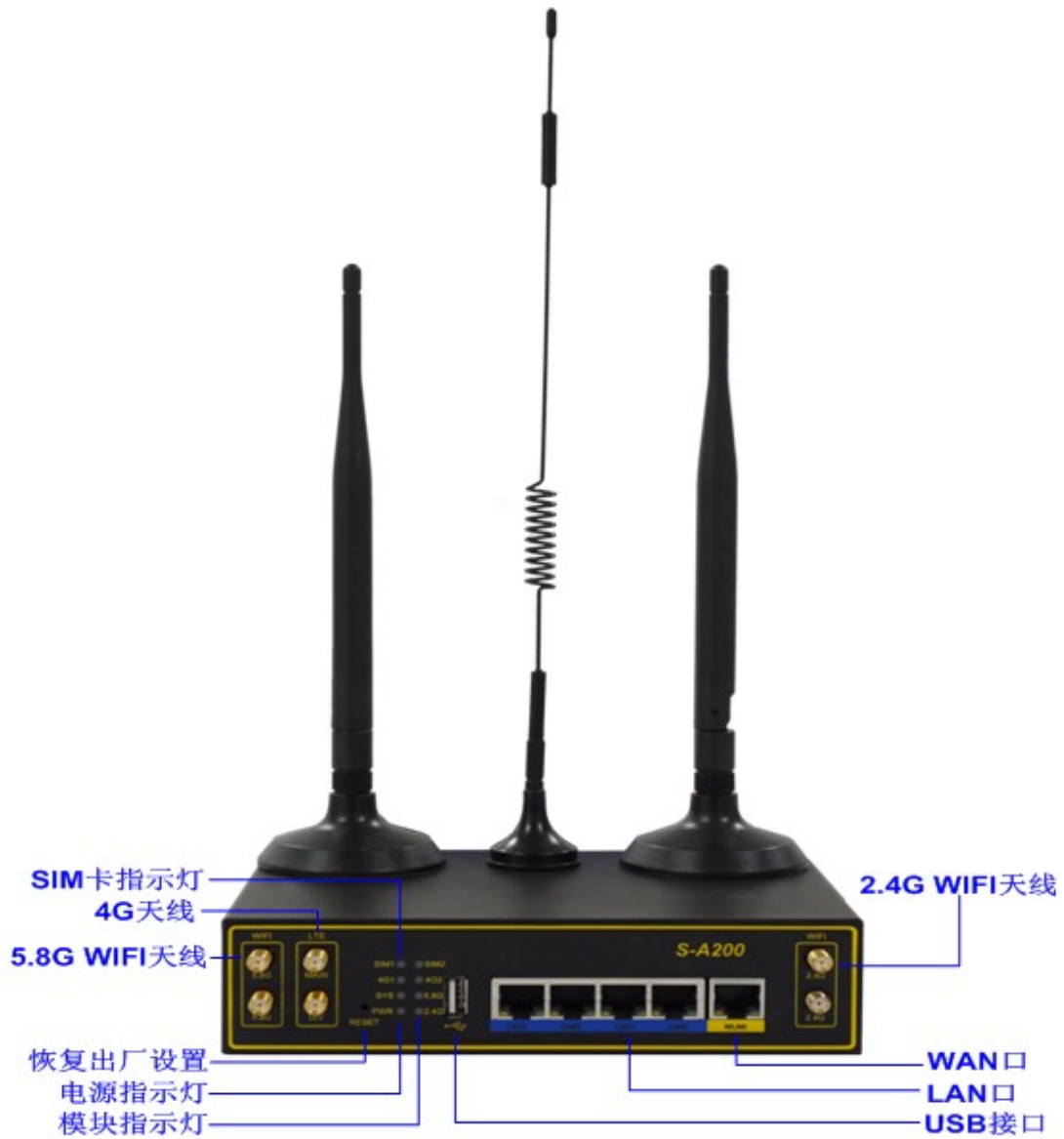
图 1-2 S-A200 前面板示意图
