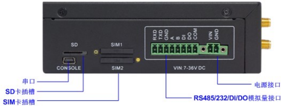
图 1-4 S-A200 侧面板示意图
